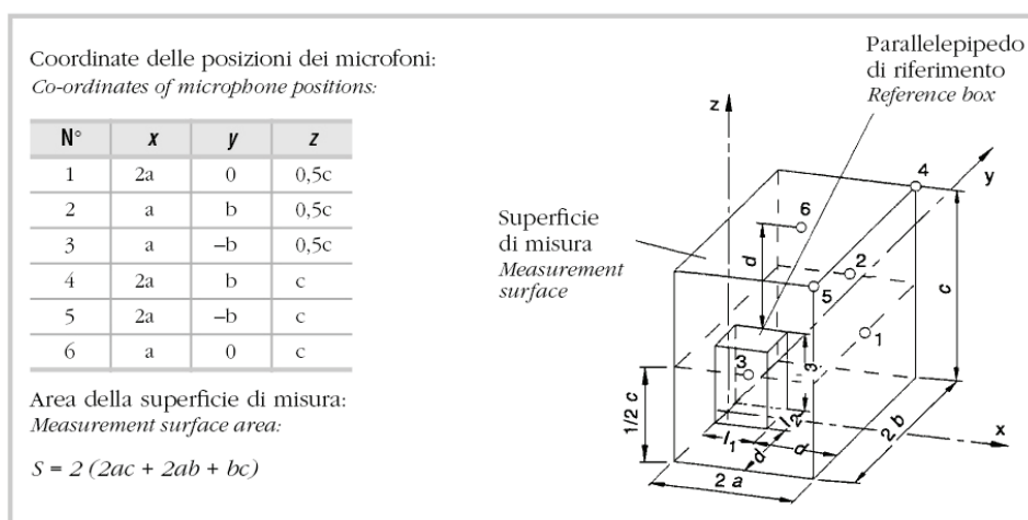
Fig. 2 Measurement surface - parallelepiped - with key microphone positions, for floor-standing appliances placed against a wall Superficie di misura - parallelepipedo - con posizioni chiave del microfono, per apparecchi posati sul pavimento contro una parete
